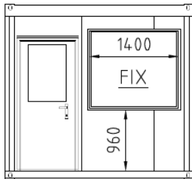
Ansicht A
