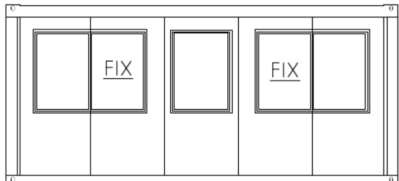
Ansicht D
