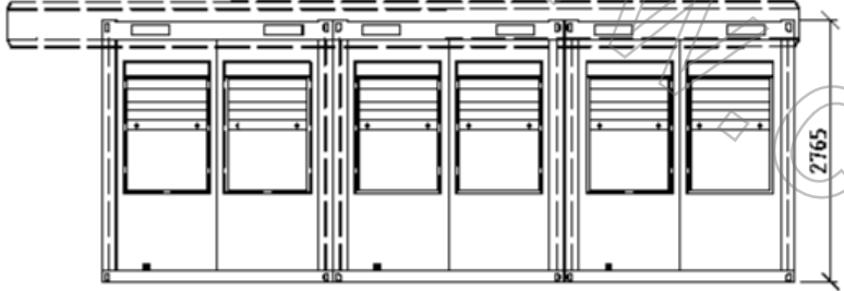
Ansicht A
