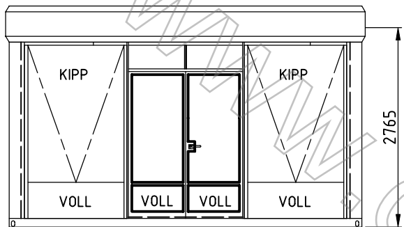
Ansicht B
