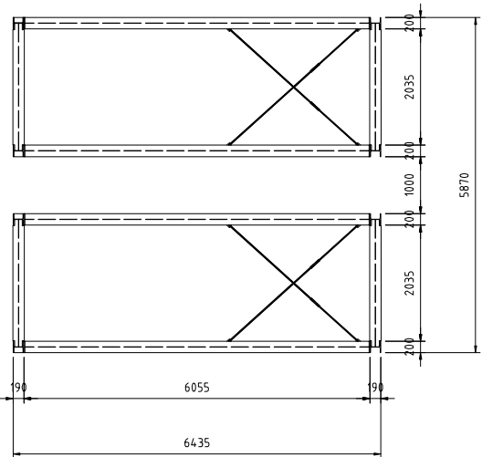
Rahmen Luftansicht:
