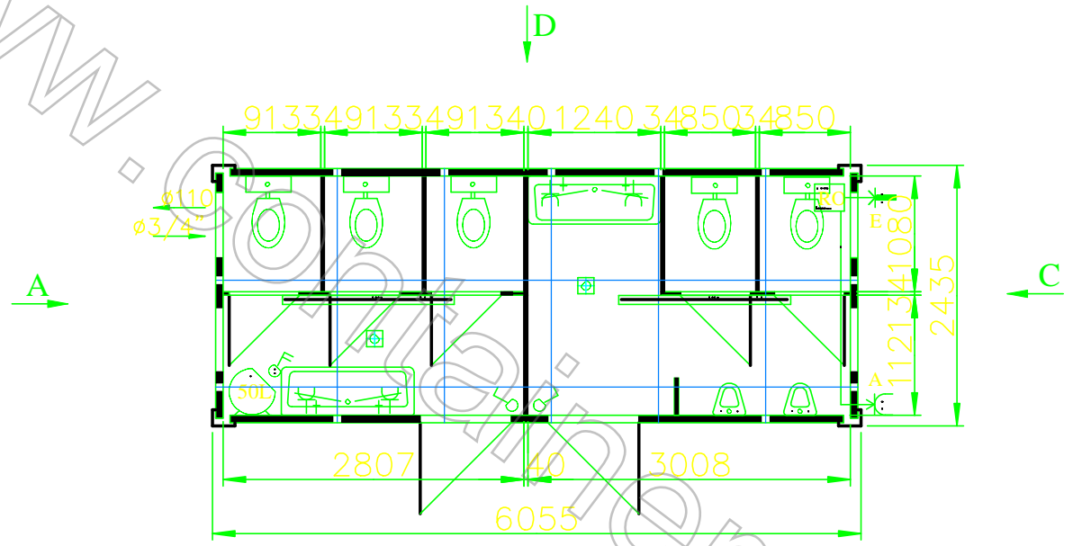
Ansicht A
