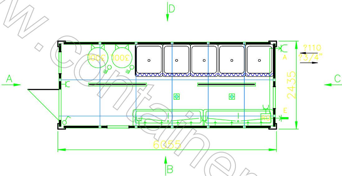
Ansicht A
