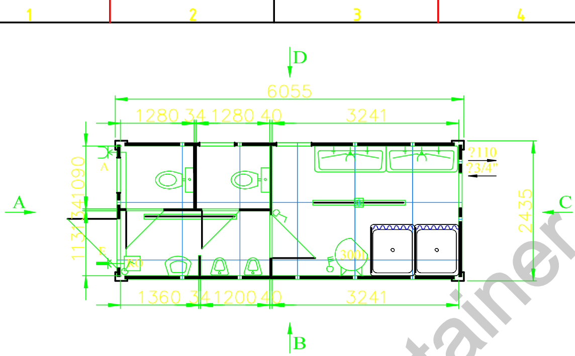
Ansicht A
