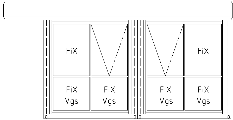
Ansicht C
