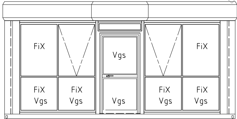
Ansicht B
